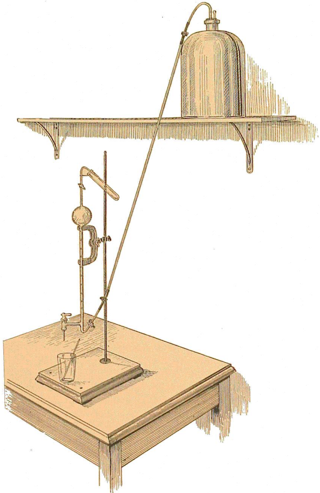
FIG. 164.—TITRATION APPARATUS.
